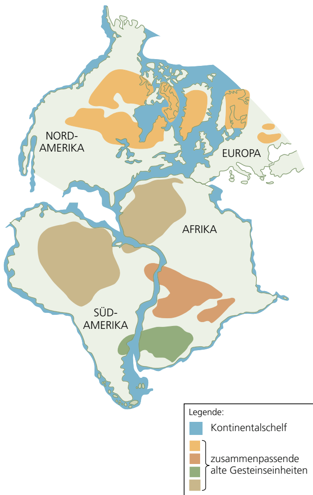
Abb. 2.1 Das puzzleartige Zusammenpassen der Kontinente, die den Atlantik umgeben, bildete die Grundlage von Alfred Wegeners Theorie der Kontinentaldrift. In seinem Buch „Die Entstehung der Kontinente und Ozeane“ führte Wegener als weiteren Beleg die Ähnlichkeit der geologischen Strukturen auf den Kontinenten beiderseits des Atlantiks an. In der Karte sind die einander entsprechenden Kristallingebiete von Südamerika und Afrika sowie von Nordamerika und Europa dargestellt (Geographische Anordnung nach Daten von E. C. Bullard; geologische Daten nach P. M. Hurley)
