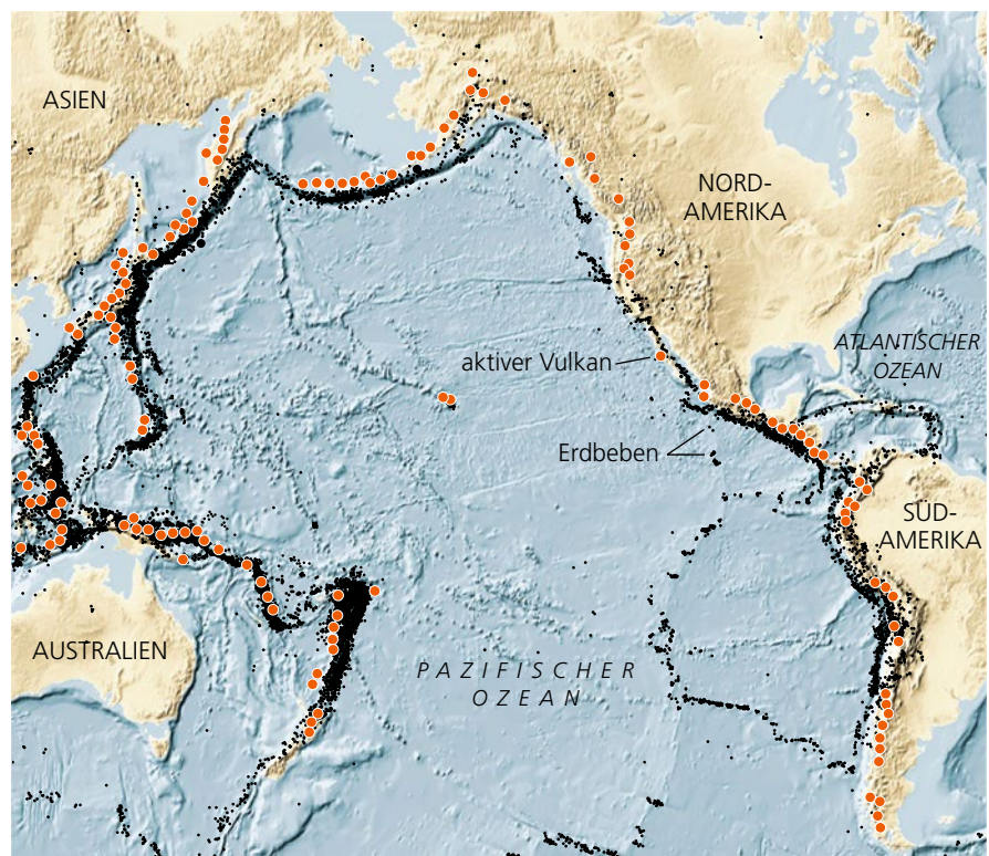
Abb. 2.6 Der „Zirkumpazifische Feuerring“ mit seinen aktiven Vulkanen ( große rote Punkte ) und häufigen Erdbeben ( schwarze Punkte ) kennzeichnet konvergente Plattengrenzen, an denen ozeanische Lithosphäre in den Erdmantel abtaucht und wieder aufgeschmolzen wird
